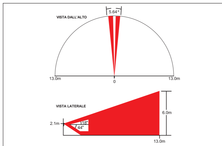
Figura 5 - Diagramma lente effetto tenda
